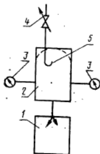
1—испытываемый насос; 2—измерительная камера; 3—измерительные преобразователи давления; 4—нагнетатель; 5—напускная трубка
