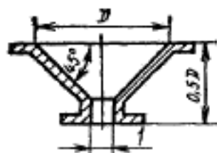
d —диаметр входного отверстия испытуемого насоса
